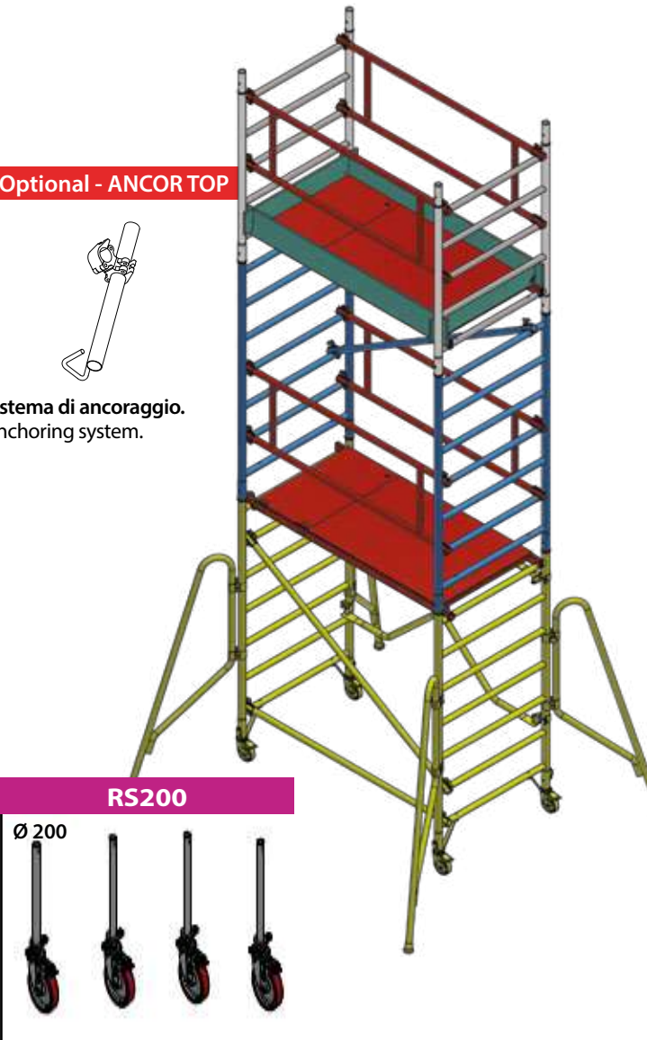
kit 4 ruote con sistema di bloccaggio. Kit with 4 scaffold wheels with lock system.
