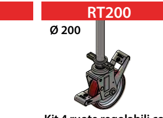
Kit 4 ruote regolabili con carico assiale quando il freno è attivo. Kit with 4 adjustable wheels. They support axial load when the brake is active.
