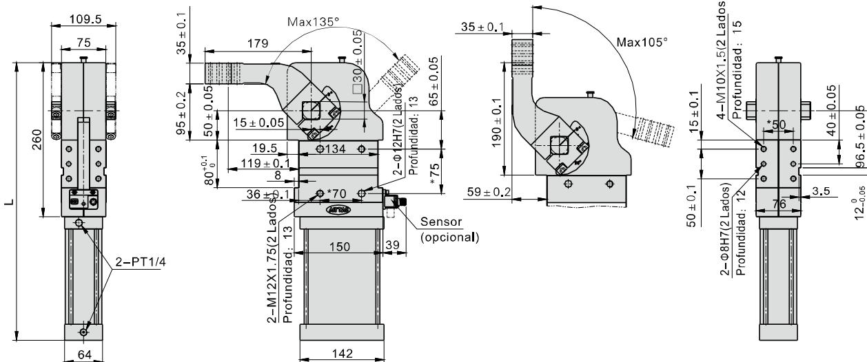
Posición de sujeción vertical
