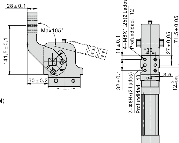
Posición de sujeción vertical
