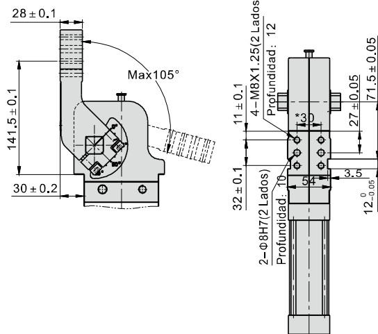
Posición de sujeción vertical
